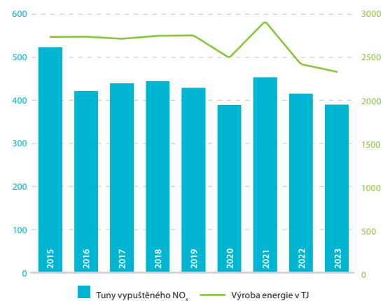
Množství \text{NO}_x vypuštěného do ovzduší v porovnání s výrobou energie
